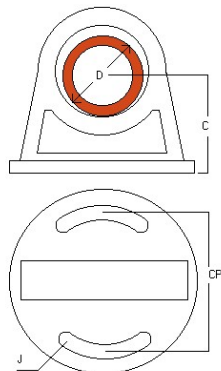
SOPORTE TUBO AISLADOR DESLIZANTE TUBO 1" A 4" - SD
