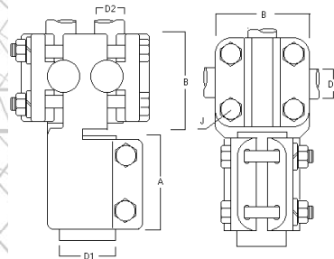
TERMINAL RECTO OTE BARRA Ø SIN HILO A 2 CABLES - WT2Y
