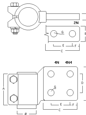
TERMINAL TE BARRA Ø SIN HILO A PALETA - WPV 2N
