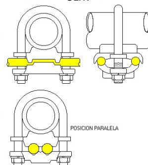
TIERRA TUBO A 2 CABLES - O2X O2XV
