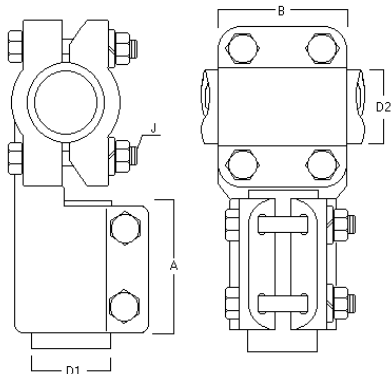
TERMINAL TE BARRA Ø CON HILO A TUBO - VXT
