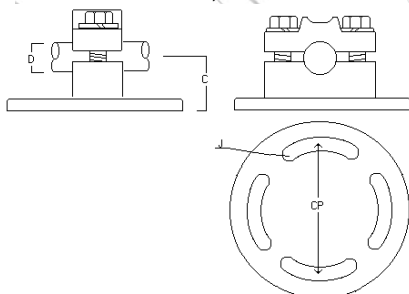
SOPORTE TUBO AISLADOR DESLIZANTE TUBO 1" A 4" - SD
