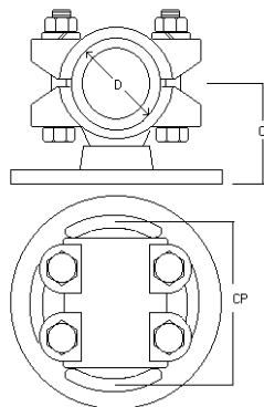
SOPORTE TUBO AISLADOR TUBO 1" A 4" - SFTR
