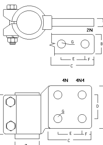
TERMINAL TE BARRA Ø CON HILO A PALETA - VPN 2N
