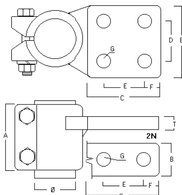
TERMINAL TE BARRA Ø CON HILO A PALETA - VPH 4N 4N4
