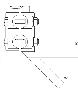
RECTO TUBO A PALETA EN ANGULO HASTA 90° - RTP90
