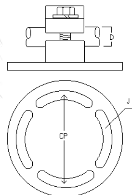
SOPORTE TUBO AISLADOR TUBO DESDE 1" A 4" - SFT
