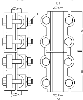
RECTO CABLE A CABLE 2 AWG A 2000 MCM - RC
