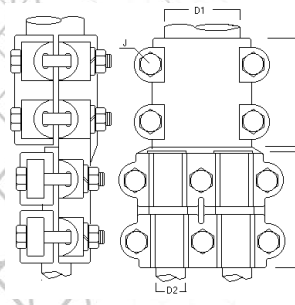
RECTO TUBO A 2 CABLES TUBO 1" A 4" CABLE 2AWG A 2000 MCM - RT2C
