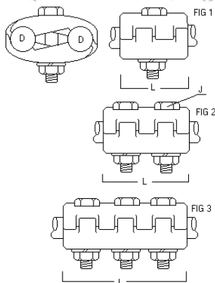
PRENSA PARALELA - I
