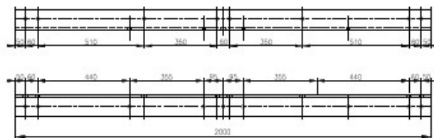
CRUCETA DE 100 x 100 x 10 x 2000 mm
