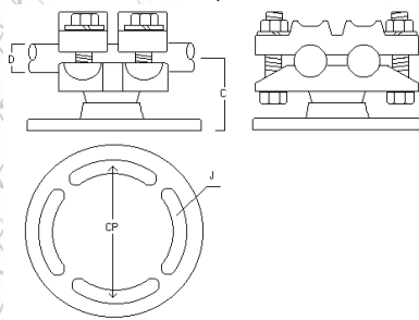
SOPORTE TUBO AISLADOR DESLIZANTE TUBO 1" A 4" - SET
