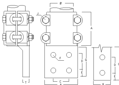
RECTO TUBO A PALETA TUBO 1" A 4" - RTP
