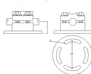
SOPORTES CABLE AISLADOR 2AWG A 2000 MCM AISLADOR 3", 5 Ó 7" - SFCR
