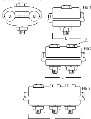
PRENSA PARALELA - IE
