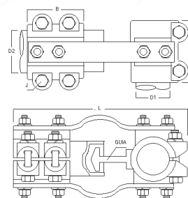
TERMINAL TE FLEXIBLE BARRA Ø CON HILO A TUBO - VXTN90
