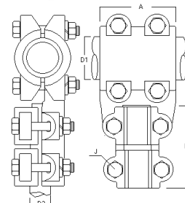
TE TUBO A PALETA TUBO - 3/4" A 4" PALETA HASTA 5" DE ANCHO TTP
