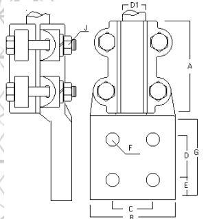
RECTO CABLE A PALETA CABLE 2AWG A 2000 MCM - RCP
