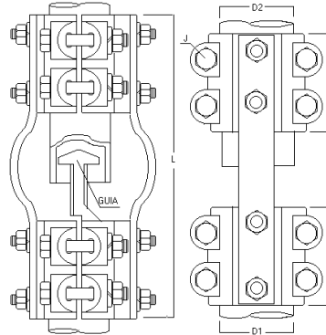
TERMINAL RECTO FLEXIBLE BARRA Ø CON HILO A TUBO - VVN
