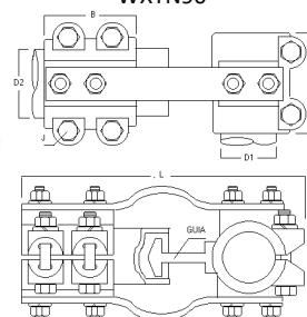
TERMINAL TE FLEXIBLE BARRA Ø SIN HILO A TUBO - WXTN90
