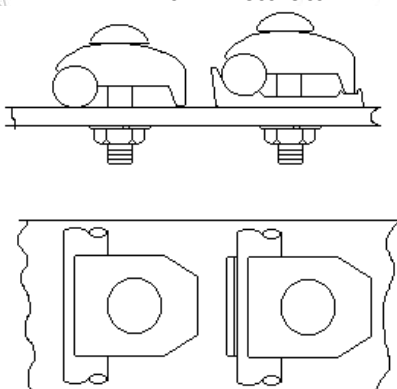
TIERRA 1 CABLE - OSS OCS
