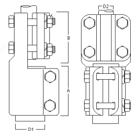
TERMINAL RECTO BARRA Ø CON HILO A CABLE - VY
