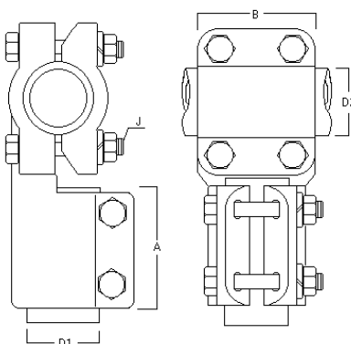
TERMINAL TE BARRA Ø SIN HILO A TUBO - WXT
