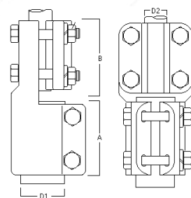
TERMINAL RECTO BARRA Ø SIN HILO A CABLE - WY
