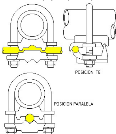
TIERRA TUBO A 1 CABLE - OXY
