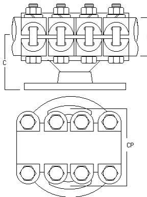
SOPORTE TUBO AISLADOR TUBO 1" A 4" - SFTE
