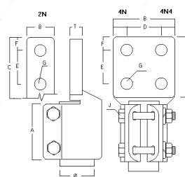
TERMINAL RECTO BARRA Ø CON HILO A PALETA - VP
