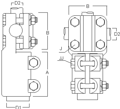
TERMINAL RECTO O TE BARRA Ø SIN HILO A CABLE - WT2Y
