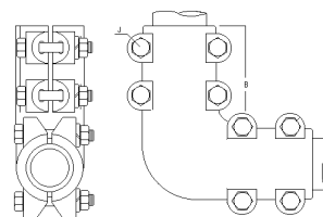
TE CURVA 90° O 45° 90° 45° - R90 R45
