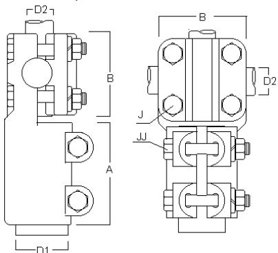
TERMINAL TE BARRA Ø CON HILO A PALETA - VPH 4N 4N4
