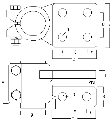
TERMINAL TE BARRA Ø SIN HILO A PALETA - WPH 4N 4N4
