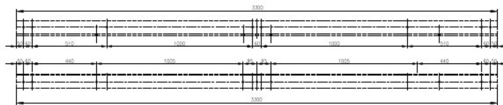
CRUCETA DE 100 x 100 x 10 x 3300 mm
