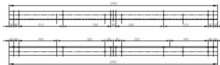
CRUCETA DE 100 x 100 x 10 x 2400 mm
