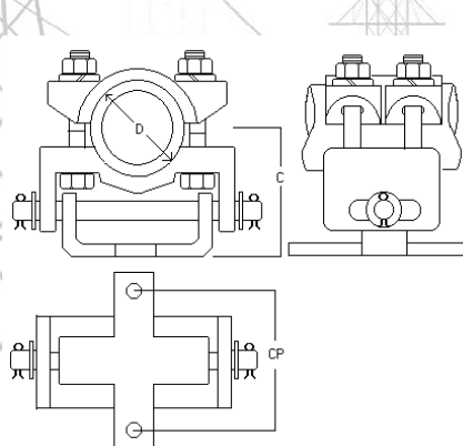
SOPORTE TUBO AISLADOR DESLIZANTE TUBO 1" A 4" - SET
