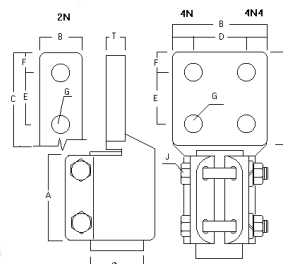
TERMINAL RECTO BARRA Ø SIN HILO A PALETA - WP
