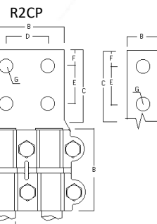
RECTO 2 CABLES A PALETA - CABLE 2AWG A 2000 MCM
