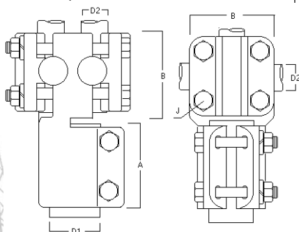
TERMINAL RECTO OTE BARRA Ø CON HILO A 2 CABLES - VT2Y
