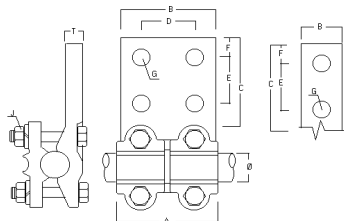
TE CABLE A PALETA CABLE 2 AWG A 2000 MCM - TCP
