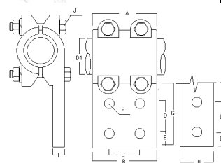
TE TUBO A PALETA TUBO - 3/4" A 4" PALETA HASTA 5" DE ANCHO TTP
