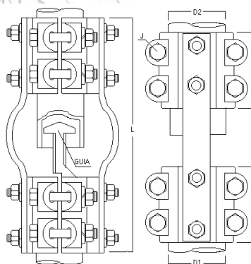
TERMINAL RECTO FLEXIBLE BARRA Ø SIN HILO A TUBO - WXN
